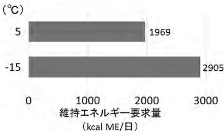
図1 環境温度と子牛のエネルギー要求
